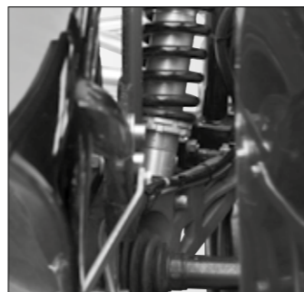
Fahrwerk: Aluminium Schräglenker und verstellbares Bilstein Gewindefahrwerk mit drei wählbaren Federn: weich, normal oder hart.
